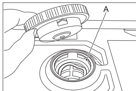
燃料口フィルタ
